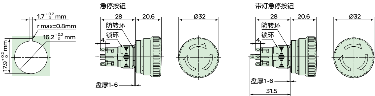
外形尺寸(适用于急停按钮)
