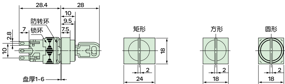
外形尺寸(适用于钥匙开关)
